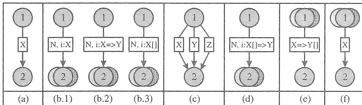
Figura 3.2 - Interações entre nodos de processamento
